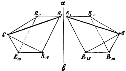
Фиг. 5. \alpha\beta —плоскость зеркала, находящаяся между энантиоморфными системами CR_I R_{II} R_{III} R_{IV} .
